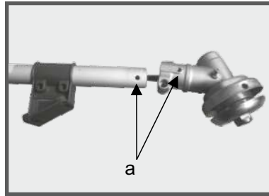
23. Соберите редуктор, как указано на рисунке. а) Два отверстия должны быть совмещены.
